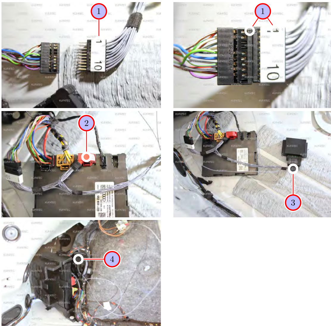
Abbildung 6: Cabrio Pro Comfort Modul anschließen
